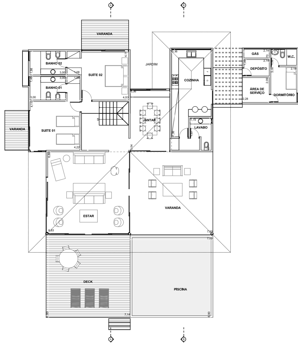
TÉRREO 1:200
